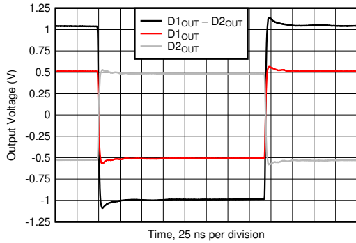
V_O step = 2\text{ V}_{PP}
